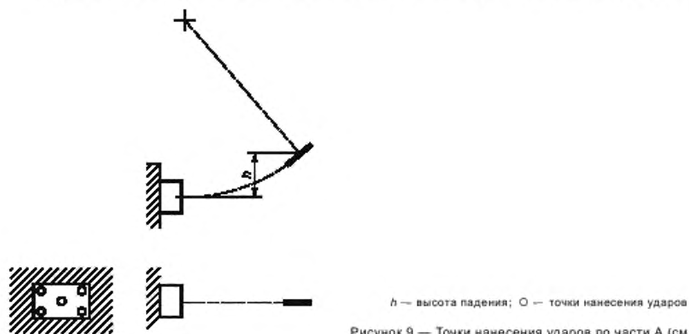
Рисунок 9 — Точки нанесения ударов по части А (см. 15.3)
