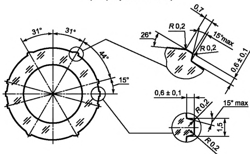
Рисунок A.7 — Шипы противоскольжения в соответствии с 4.2
