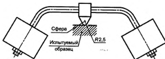
Рисунок 1 – Установка для испытания на теплостойкость
