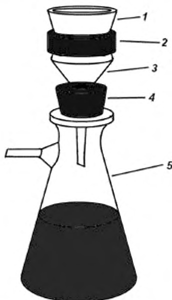
1 — тигель Гуча; 2 — резиновая соединительная трубка; 3 — фильтровальная трубка; 4 — неопределенная пробка; 5 — фильтровальная толстостенная колба
