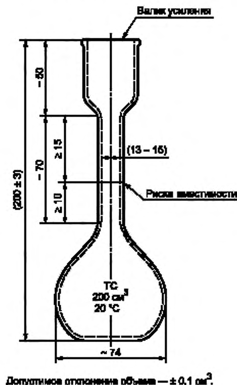
Рисунок 3 — Колба Кольрауша
