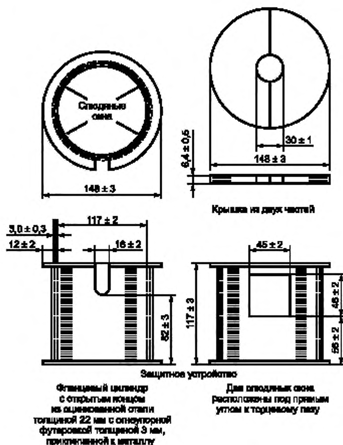
Рисунок 3 — Защитное устройство
