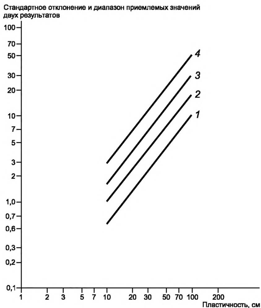
Рисунок 2 — Данные прецизионности
