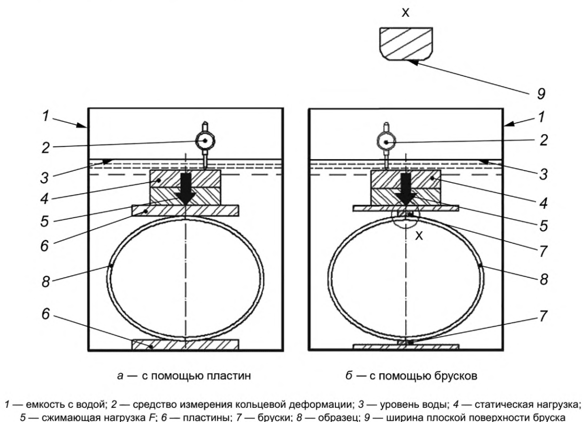
Рисунок 1 — Схемы нагружения образцов
