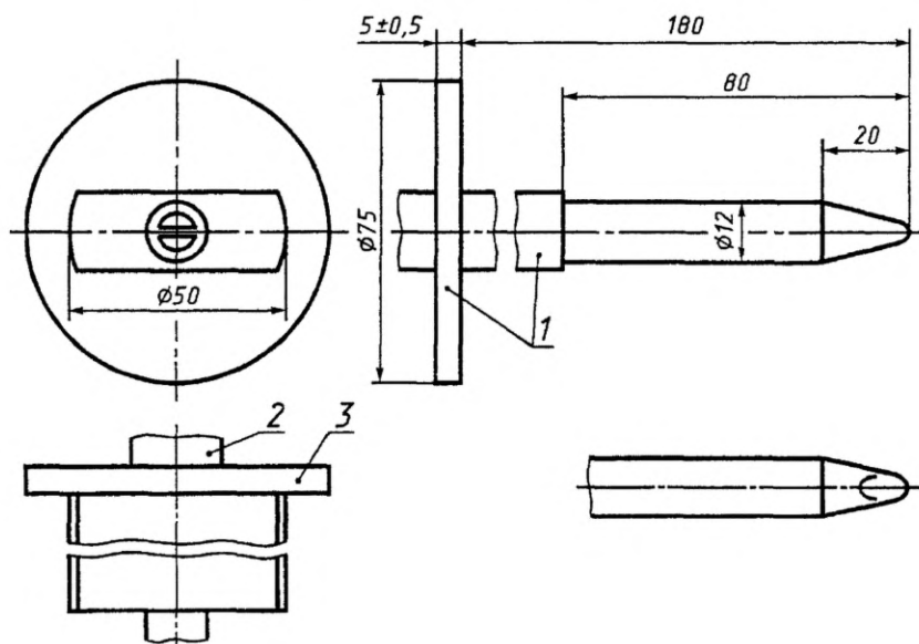
Рисунок Г.1 — Шарнирный испытательный палец
