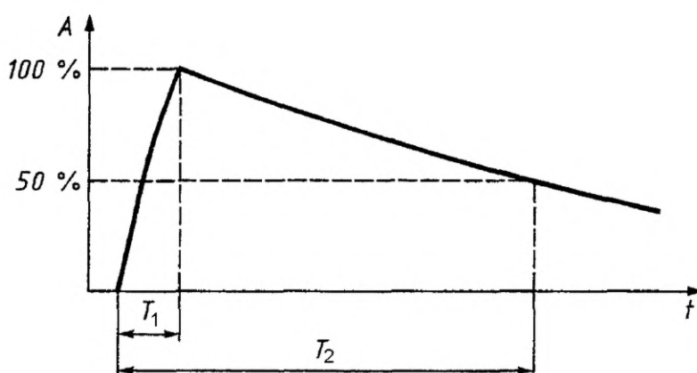
Рисунок Е.1 — Схема для испытания импульсным перенапряжением
