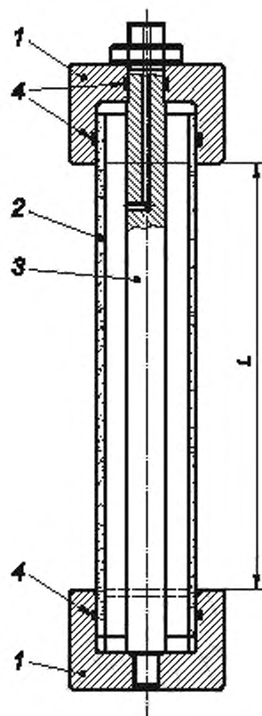
1 — торцевая заглушка; 2 — образец; 3 — штанга; 4 — эластомерный уплотнитель; L — длина образца между заглушками
