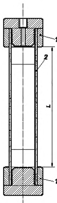
1 — торцевая заглушка; 2 — образец; L — длина образца между заглушками
