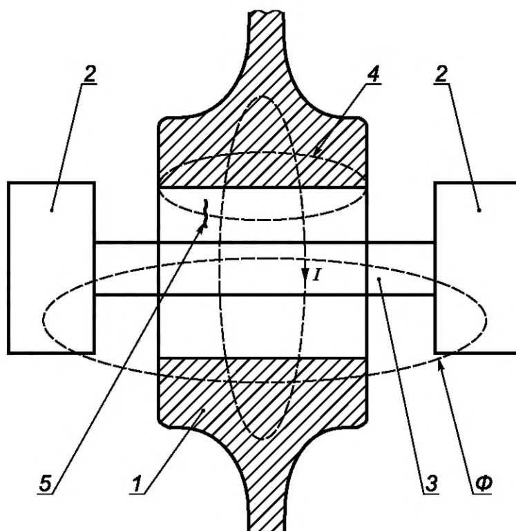
1 — цельнокатаное колесо; 2 — электромагнит; 3 — проводник; 4, \Phi — магнитные потоки; 5 — дефект; I — индуцированный ток
