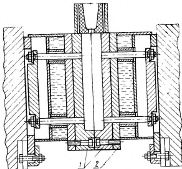
1—кокиль; 2—плита охлаждающая.
