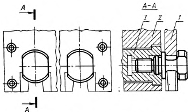
1—плита из чугуна; 2—плата переходника; 3—фланец переходника
