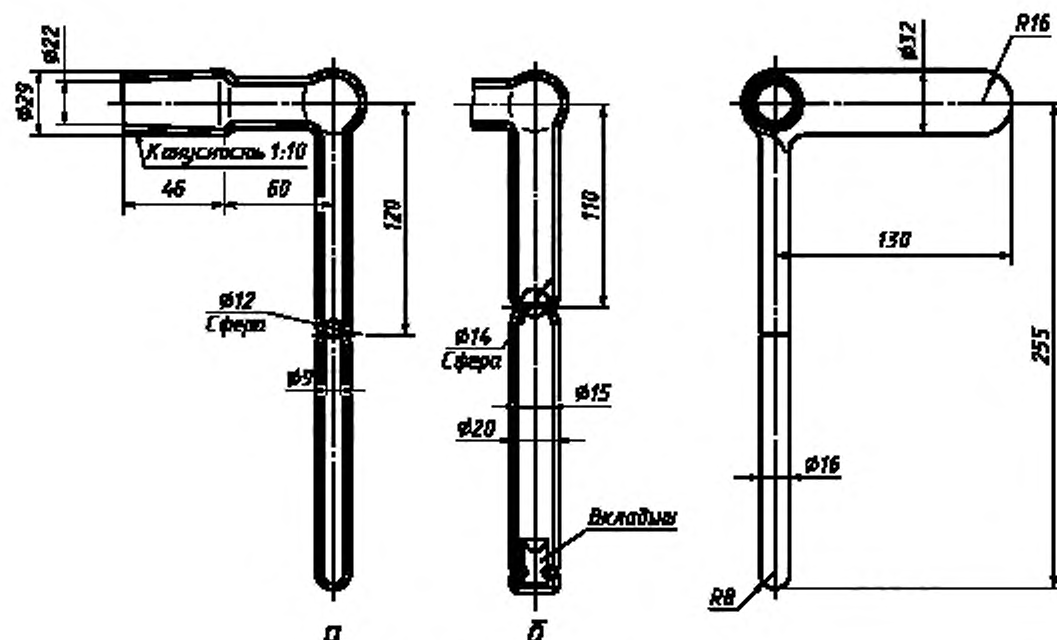
а — трубка без вкладыша; б — трубка с вкладышем
