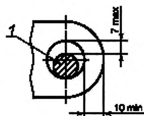
Рисунок 8 — Установка задвижки с проушинами под навесной замок
