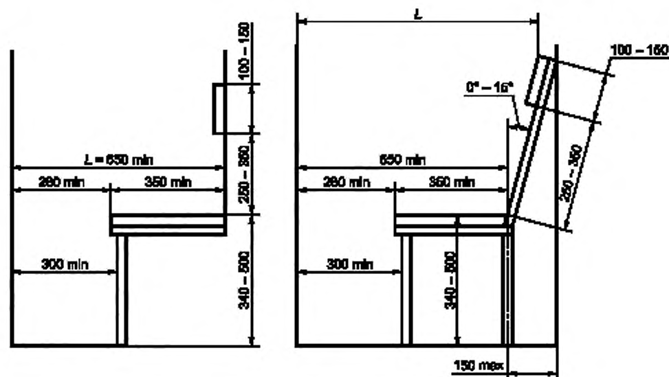
Рисунок 3 — Размеры сидений разных типов и размеры отсека для задержанных с одним рядом сидений
