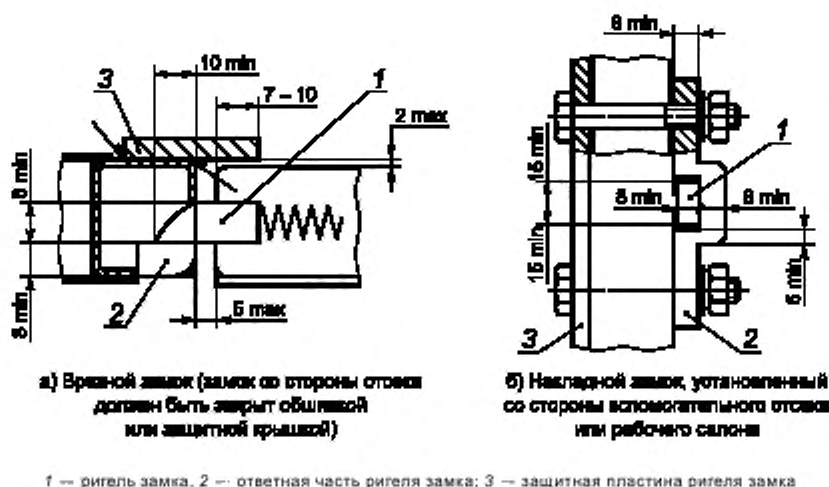
Рисунок 7 — Варианты установки замков дверей отсека для задержанных
