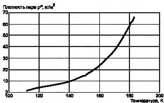
Рисунок А.3 — Плотность насыщенного пара метана
