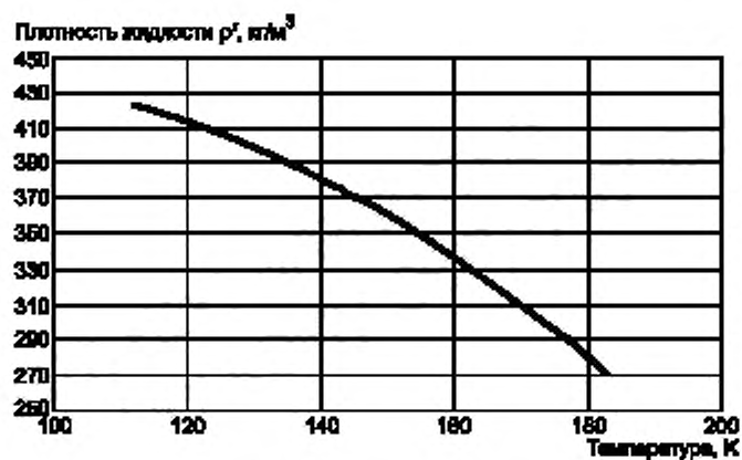
Рисунок А.2 — Плотность жидкого метана
