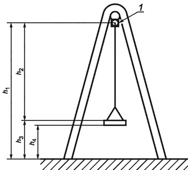
Рисунок 5 — Размеры по высоте
