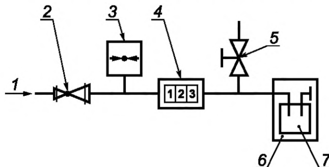
1 — вход испытательного газа; 2 — регулятор давления; 3 — манометр; 4 — измерительный прибор; 5 — выпускной клапан; 6 — печь; 7 — кран, подлежащий испытанию в частично открытом положении
