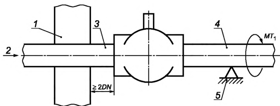
1 — зажим для труб; 2 — испытательное давление; 3 — труба 1; 4 — труба 2; 5 — поддерживающая труба
