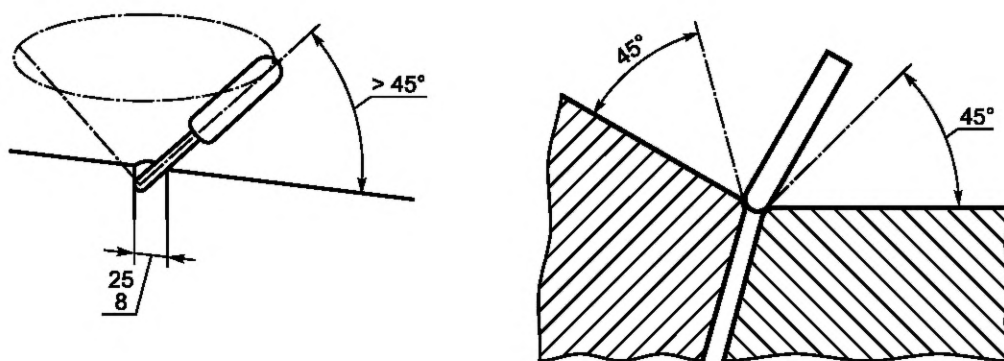
Рисунок D.11 — Круговое движение стержня-пальца диаметром 8 мм
