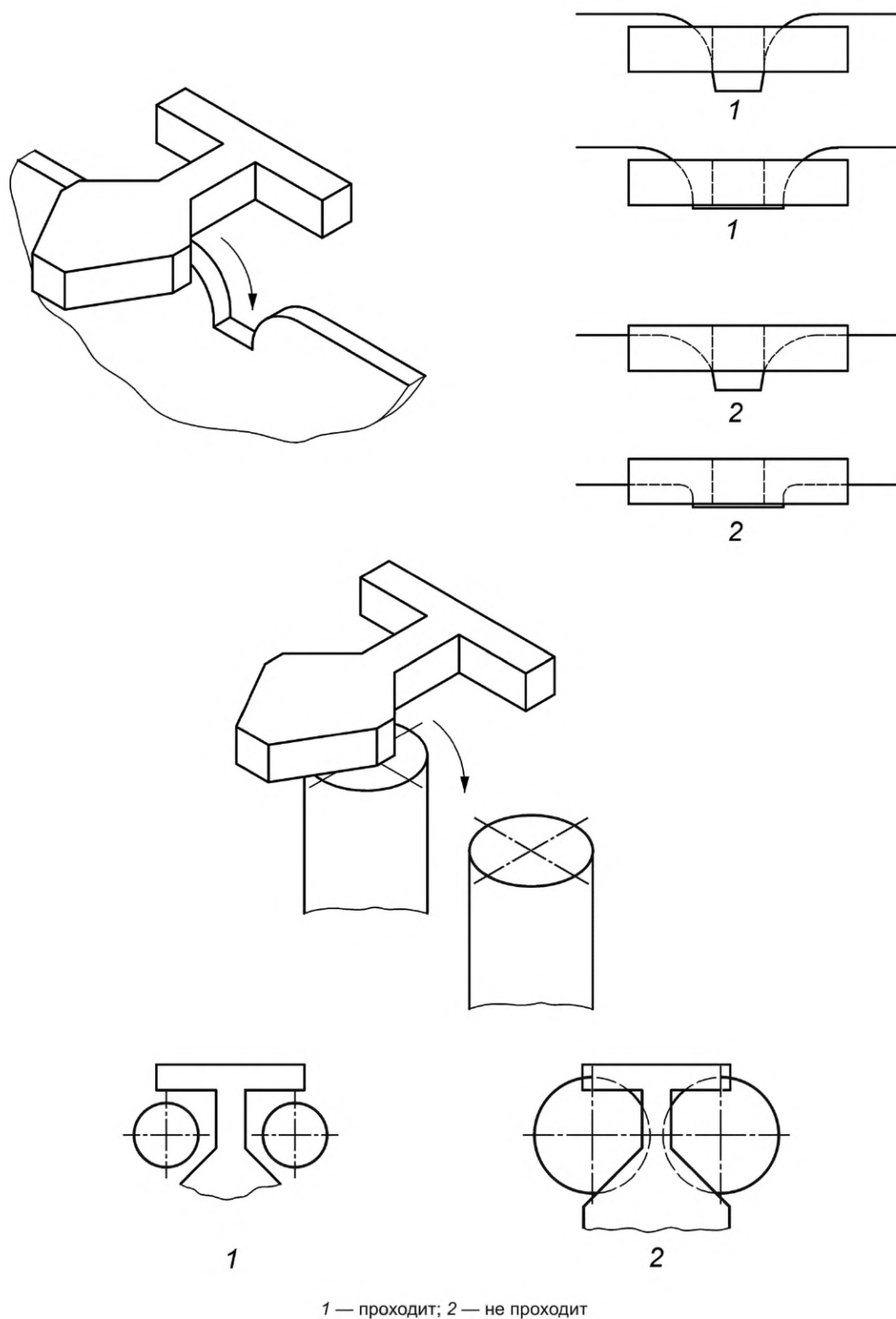
Рисунок D.3 — Способ применения части шаблона «В»
