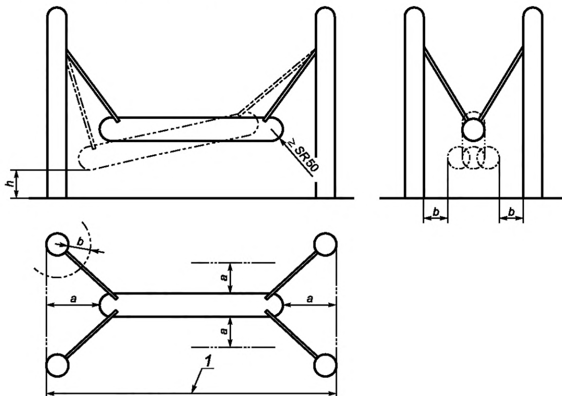
Рисунок 25 — Пример раскачивающегося бруса
