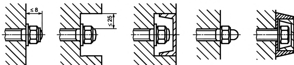
Рисунок 11 — Примеры защиты гаек и болтов
