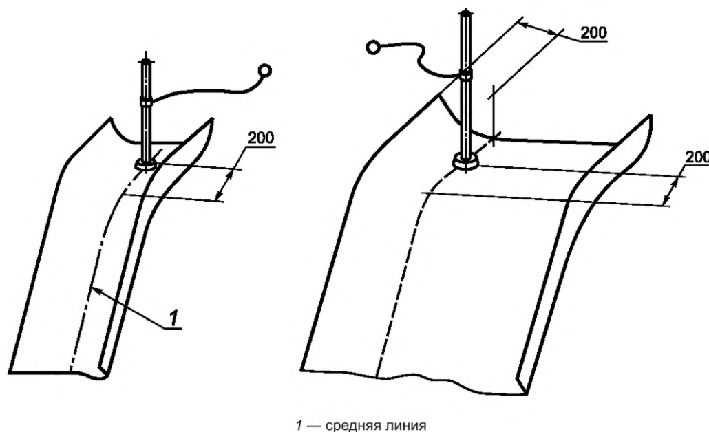
Рисунок D.8 — Расположение испытательного устройства на горках
