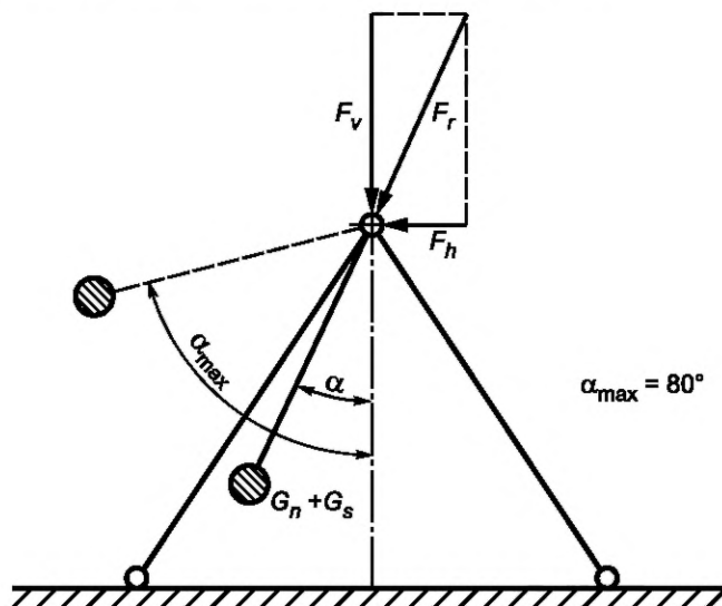
Рисунок В.2 — Нагрузки, действующие на качели
