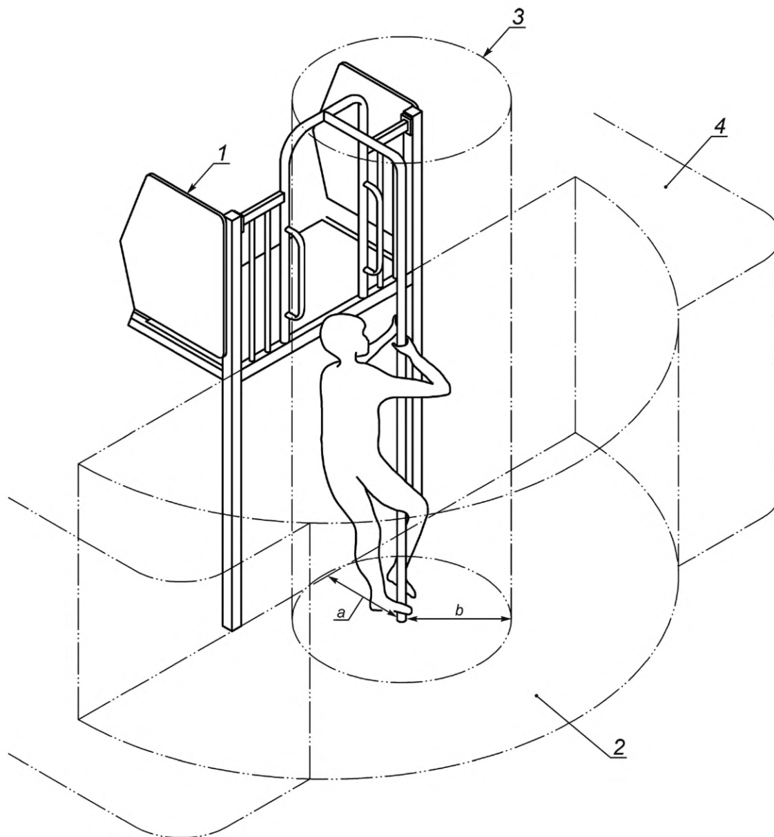
1 — пространство оборудования; 2 — пространство падения шеста; 3 — свободное пространство шеста; 4 — пространство падения платформы; a — минимальное расстояние шеста (см. 4.2.8.3); b — радиус свободного пространства (см. 4.2.8.2.3)
