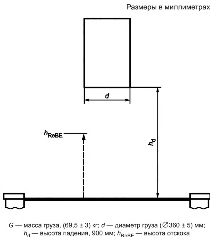
Рисунок D.14 — Испытание на определение высоты отскока на прыжковом устройстве
