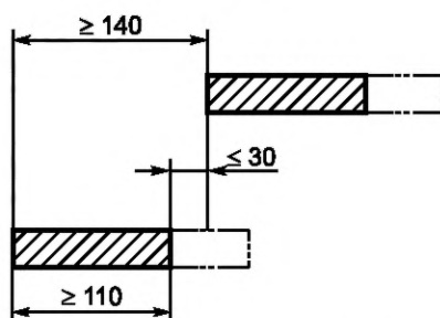
Рисунок 22 — Проекция и глубина ступени
