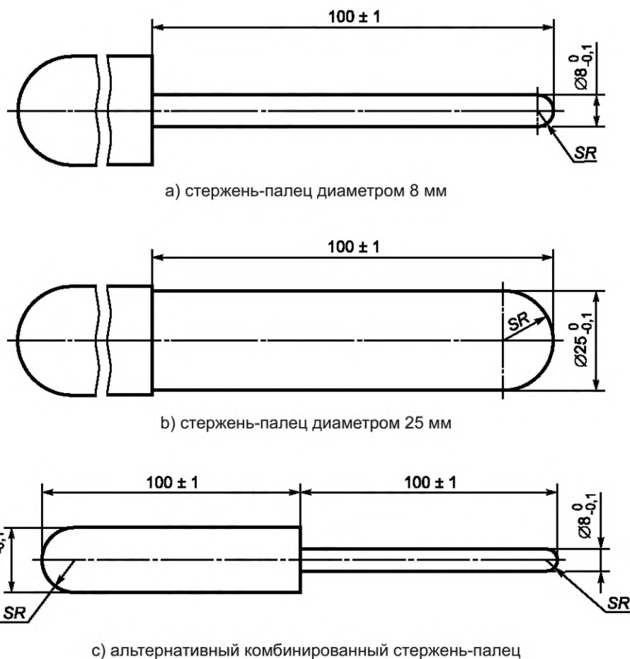
Рисунок D.10 — Стержни-пальцы
