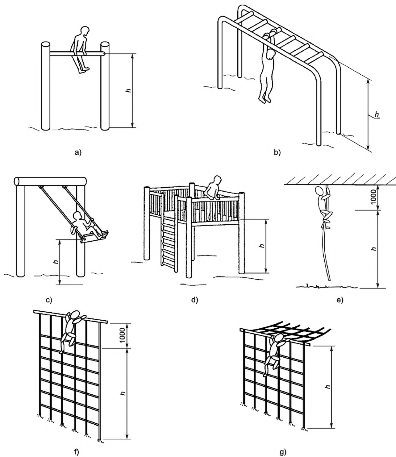
Рисунок 14 — Примеры, иллюстрирующие высоту свободного падения
