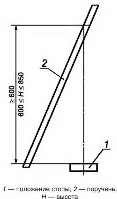
Рисунок 9 — Руководство по измерению высоты поручня над положением стопы
