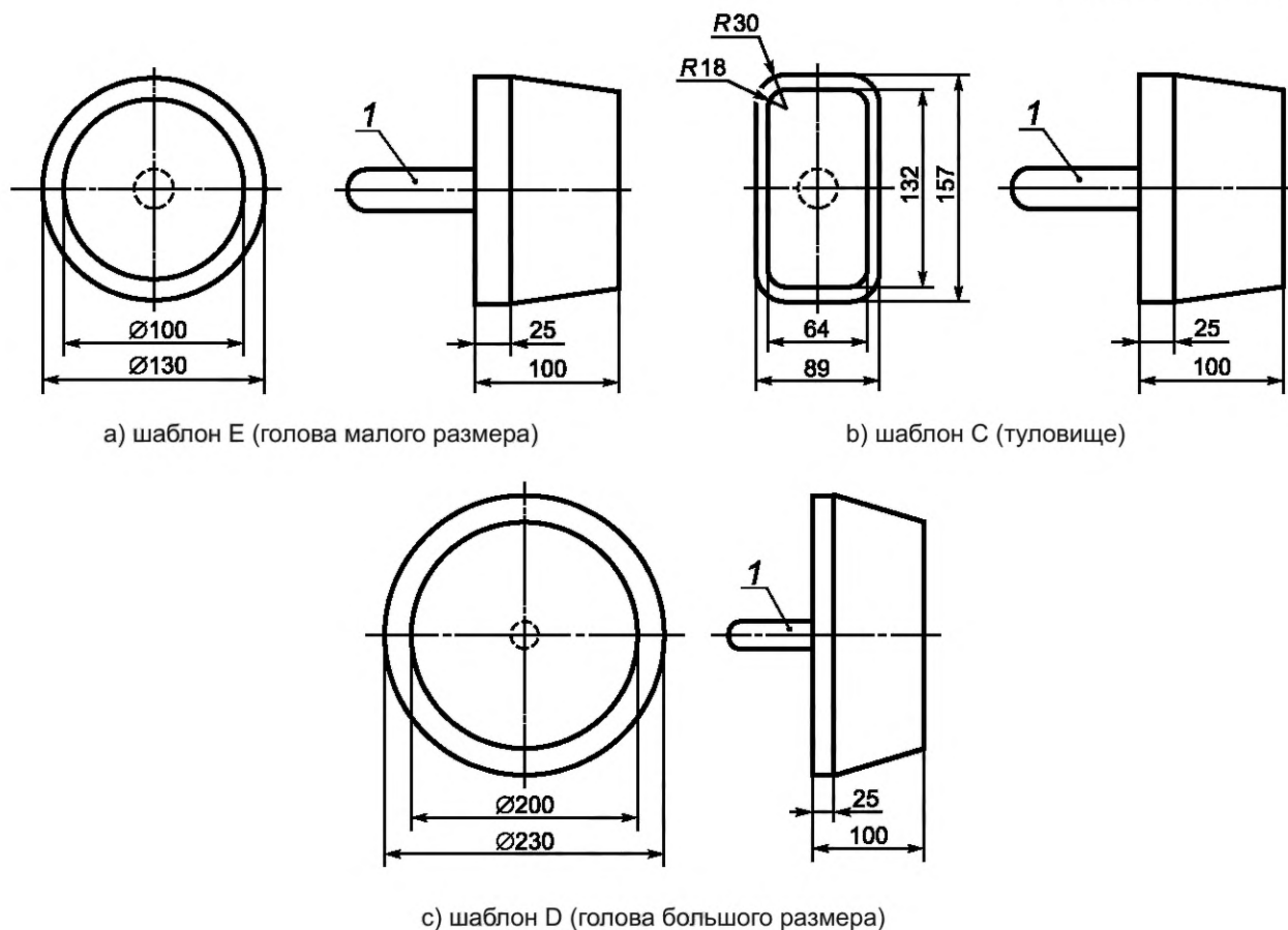
Рисунок D.1 — Шаблоны для определения мест заземления головы и шеи в полностью замкнутых проемах
