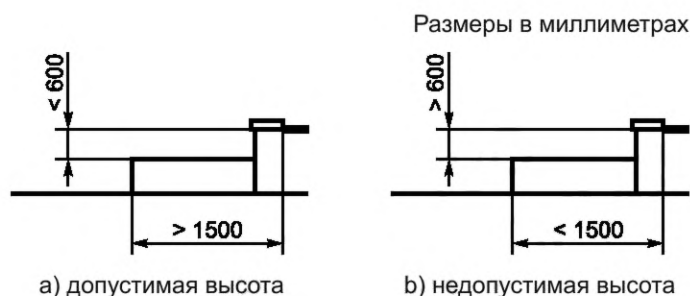
Рисунок 26 — Допустимая и недопустимая высоты прыгательной поверхности
