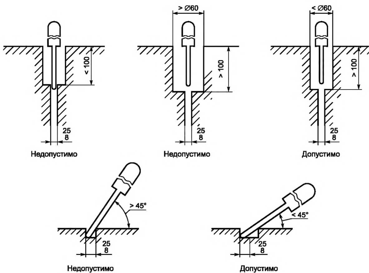
Рисунок D.12 — Возможность прохождения стержня-пальца
