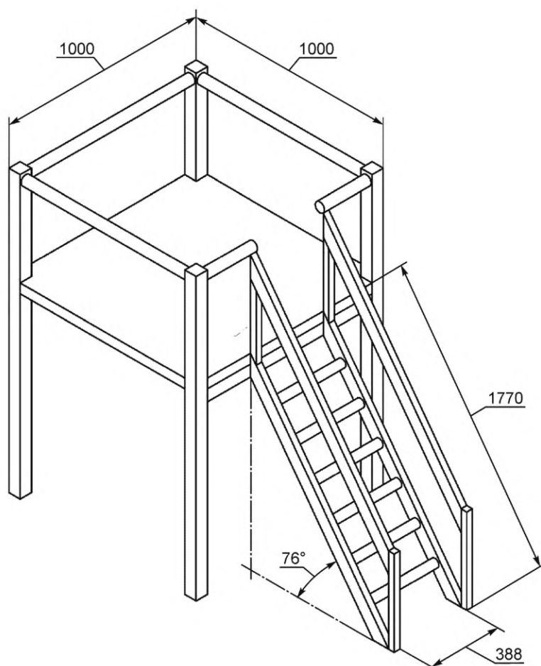
Рисунок В.1 — Платформа с лестницей
