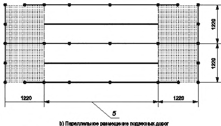
Рисунок 4 — Подвесные дороги — типовые схемы
