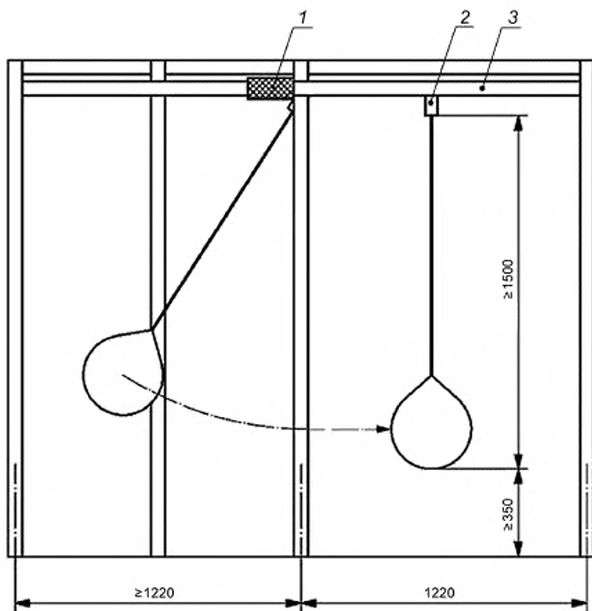
1 — стопор; 2 — каретка; 3 — направляющая подвесной дороги
