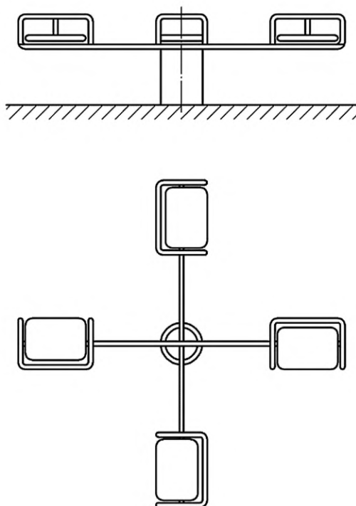
Рисунок 1 — Пример карусели типа А (вращающиеся сиденья)
