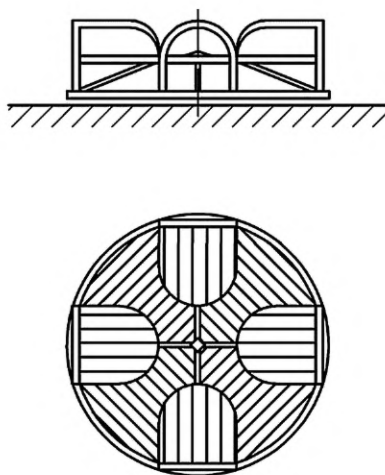
Рисунок 2 — Пример карусели типа В (классическая карусель)
