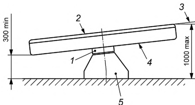
1 — подшипник; 2 — верхняя поверхность; 3 — наклон; 4 — нижняя поверхность; 5 — опора/фундамент
