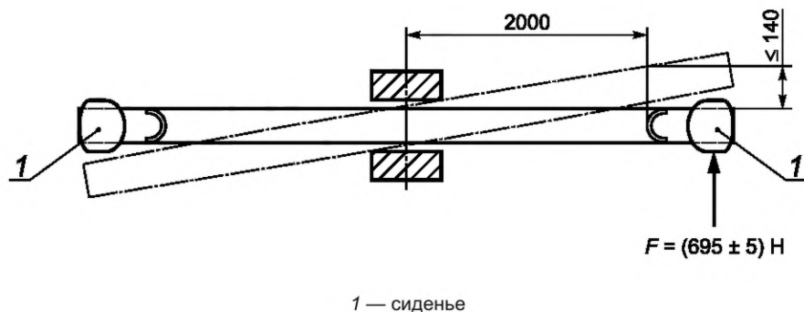
Рисунок 11 — Отклонения в горизонтальной плоскости качалок-балансиров типа 1
