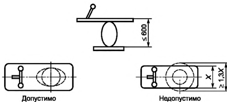
Рисунок 10 — Прикрытие основания
