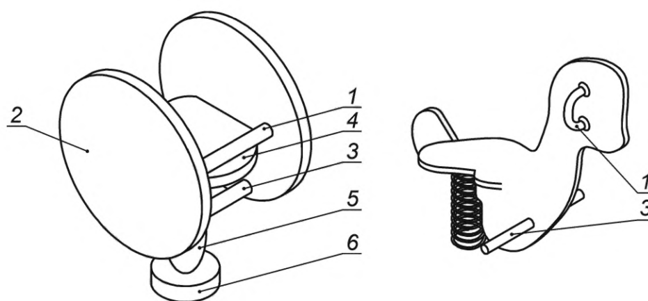
а) Качалка
