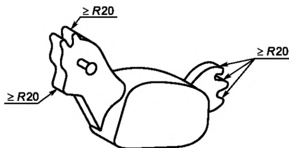
Рисунок 8 — Форма профиля со скругленными углами
