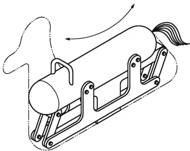
Рисунок 5 — Пример шатунной качалки (тип 4)
