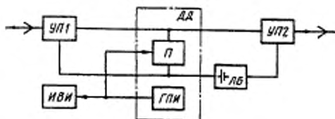
Схема измерения при дроблении минусовой значащей посылки
