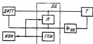
Схема измерения при дроблении бестоковой значащей посылки
