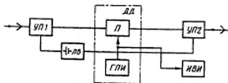
Схема измерения при дроблении плюсовой значащей посылки
