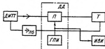
Схема измерения при дроблении токовой значащей посылки
