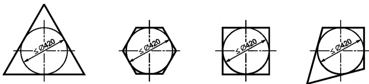
Рисунок 4 — Базовые размеры ячейки пространственной игровой сети
