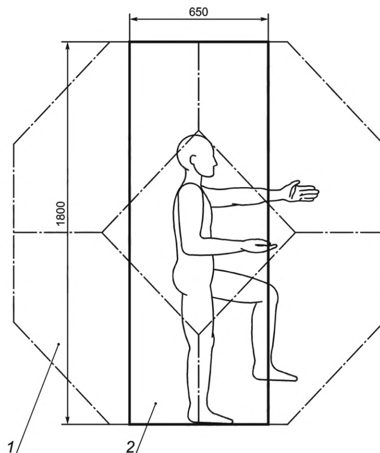
1 — пространственная игровая сеть; 2 — цилиндрический шаблон
