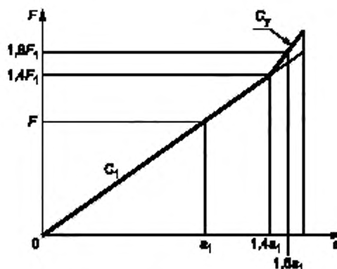
Рисунок 3 — Силовые характеристики пружинных комплектов ступени РП с работающим упругим упором ( K_{КЗ} > 1,6 )
