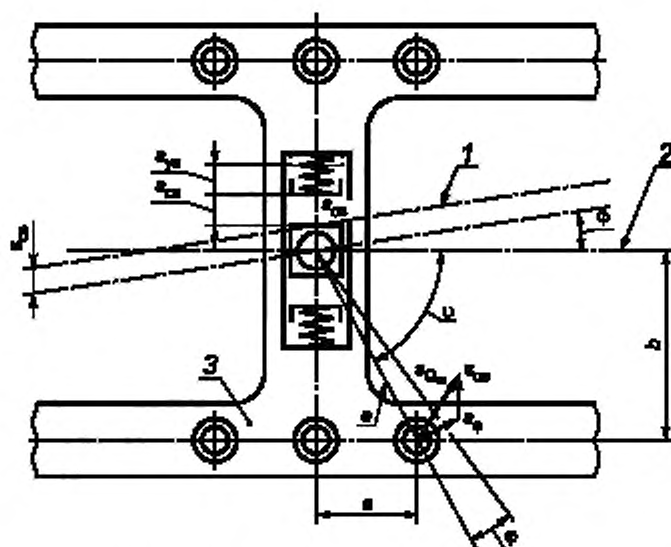
1 — ось кузова при повороте и отnose. 2 — продольная ось кузова; 3 — рама тележки
