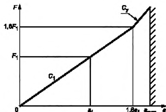
Рисунок 2 — Силовые характеристики пружинных комплектов ступени РП с наличием упругого упора ( K_{\text{кз}} > 1,6 )
