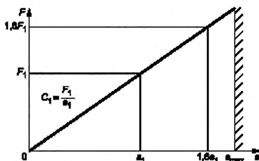
Рисунок 1 — Силовые характеристики пружинных комплектов ступени РП без упругого упора ( K_{\text{кз}} > 1,6 )
