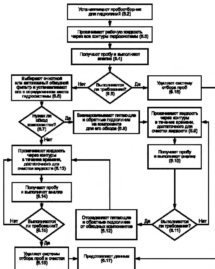
Рисунок 1 — Блок-схема, отражающая процедуру оценки чистоты собранной гидросистемы
