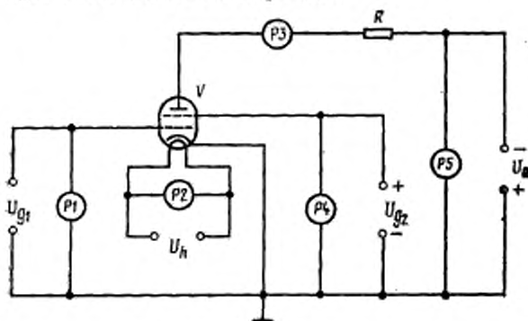
P4, P5, P1, P2 —приборы для измерения постоянного (переменного) напряжения; P3 —прибор для измерения тока;
