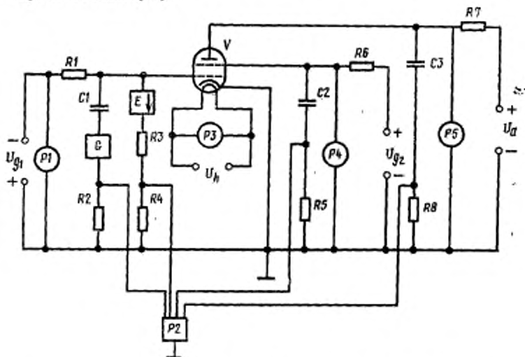
C_1 —разделительный конденсатор; C_2, C_3 —накопительные конденсаторы; E —электровакуумный или полупроводниковый диод; G —генератор импульсов; P_1, P_3, P_4, P_5 —приборы для измерения постоянного (переменного) напряжения; P_2 —электронный осциллограф; R_1 —ограничительный резистор; R_2, R_3, R_4 —измерительные резисторы; R_5, R_8 —зарядные резисторы; R_6, R_7 —зарядные резисторы; V —испытываемая лампа.
