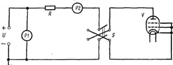
P1 —прибор для измерения постоянного напряжения; P2 —прибор для измерения постоянного тока; R —защитный резистор; S —переключатель; V —испытуемая лампа
