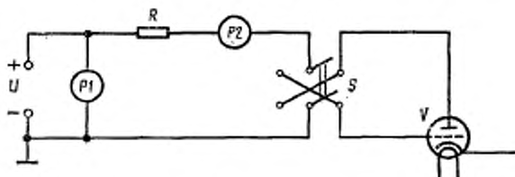
P1 —прибор для измерения постоянного напряжения; P2 —прибор для измерения постоянного тока; R —защитный резистор; S —переключатель; V —испытуемая лампа
