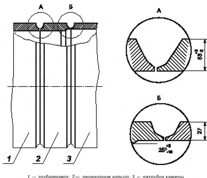
Рисунок 4 — Вариант соединения камеры при помощи переходного кольца
