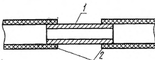
1—металлическая трубка; 2—трубопровод из изоляционного материала.
