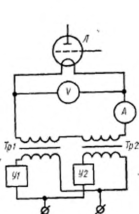
А—амперметр; V—вольтметр; Л—испытываемая лампа; Tr1, Tr2—трансформаторы напряжения накала; U1, U2—прерыватели напряжения накала
