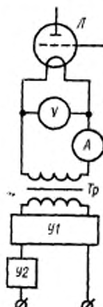
А—амперметр; V—вольтметр; Л—испытываемая лампа; Tr—трансформатор напряжения накала; U1—ограничительное устройство (регулятор напряжения); U2—прерыватель напряжения
