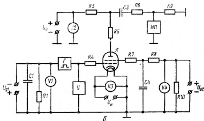
Электрическая схема испытания:
