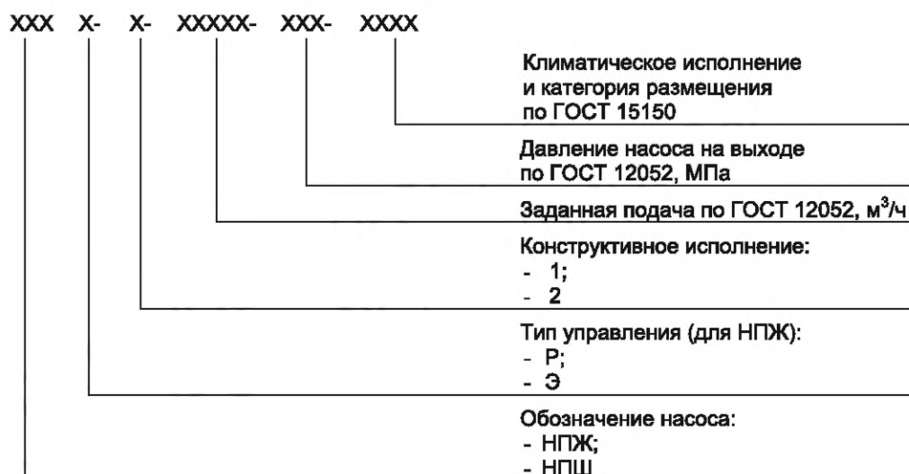
Рисунок 1 — Схема условного обозначения НПЖ и НПШ
