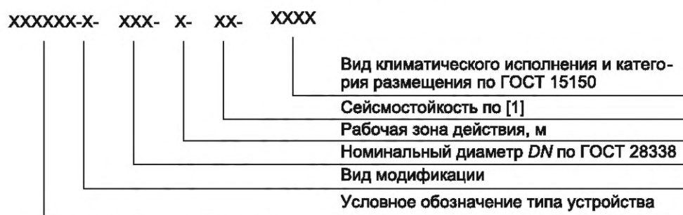
Рисунок 1 — Схема условного обозначения сливо-наливных устройств нефти/нефтепродуктов
