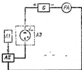
A2—устройство стабилизации длины светящегося столба; A1—фотоприемник; VL—испытуемый индикатор; A3—термокамера; G—источник напряжения постоянного тока; PA—измеритель тока.
