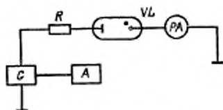
А—устройство измерения длины светящегося столба; G—регулируемый источник постоянного напряжения; R—резистор; VL—испытываемый индикатор; PA—измеритель тока.
