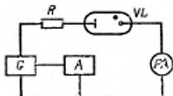
А—устройство установки фиксированной длины светящегося столба индикатора; G—регулируемый источник постоянного напряжения; R—резистор; VL—испытываемый индикатор; PA—измеритель тока
