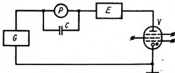
P — измеритель постоянного тока; C — конденсатор; V — испытываемый тиратрон; G — источник напряжения; E — элемент цепи анода
