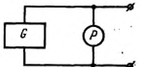
G — источник управляющего напряжения; P — измеритель напряжения
