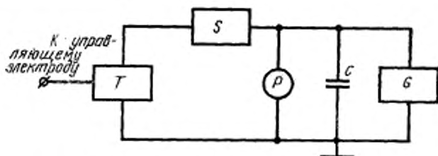
С — накопительный конденсатор; Р — измеритель напряжения; Т — импульсный трансформатор; S — коммутационное устройство; G — источник напряжения
