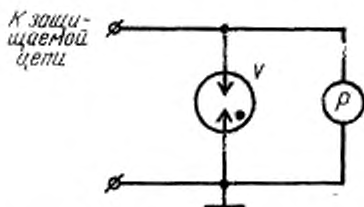
P — измеритель постоянного напряжения, V — испытываемый разрядник
