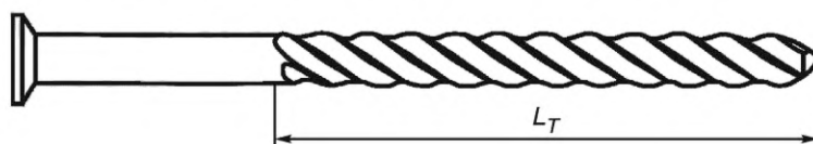
Рисунок А.3 — Схематическое представление измерения длины резьбы
