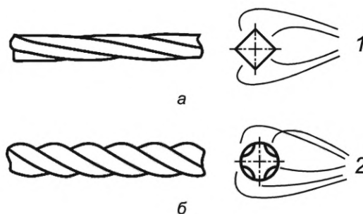
а — крученный стержень из квадратной проволоки; б — стержень со спиралевидной резьбой; 1 — четыре рифли; 2 — пять рифлей
