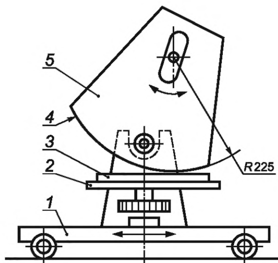
1 — площадка; 2 — стол; 3 — образец; 4 — шлифовальная шкурка; 5 — рабочий элемент
