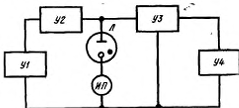
ИП — измеритель тока; Л — испытуемый стабилитрон; У1 — регулируемый источник постоянного напряжения; У2 — стабилизатор тока; У3 — делитель напряжения; У4 — потенциометр постоянного тока.
