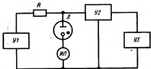
R —резистор; ИП —измеритель тока; Л —испытываемый стабилитрон; U1 —регулируемый источник постоянного напряжения; U2 —делитель напряжения; U3 —потенциометр постоянного тока.
