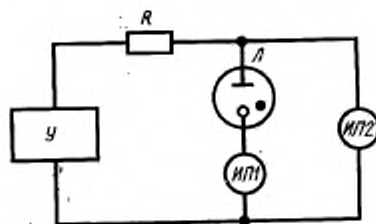
R —резистор; ИП1 —измеритель тока; ИП2 —измеритель напряжения; Л —испытуемый стабилитрон; U —регулируемый источник постоянного напряжения
