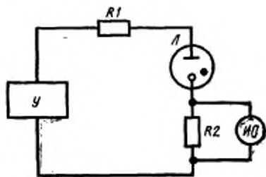
R1 , R2 —резисторы; ИП—измеритель напряжения; L —испытываемый стабилитрон; U —источник постоянного напряжения.
