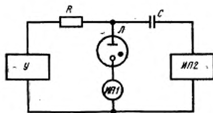
R —резистор; C —конденсатор; ИП1 —измеритель тока; ИП2 —электронный милливольтметр; Л —испытываемый стабилитрон; U —регулируемый источник постоянного напряжения.
