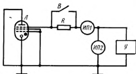
R — резистор; B — выключатель; ИП1 — измеритель тока; ИП2 — измеритель напряжения; Л — испытываемый тиратрон; У — регулируемый источник постоянного напряжения
