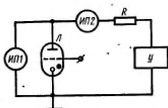
R — резистор; ИП1 — измеритель напряжения; ИП2 — измеритель тока; Л — испытуемый тиатрон (газотрон); U — регулируемый источник постоянного напряжения
