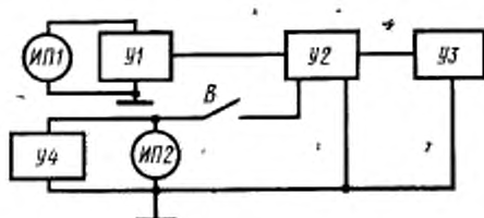
В —выключатель; ИП1 , ИП2 —измерители напряжения; У1 —регулируемый источник постоянного напряжения; У2 —устройство коммутации и испытуемый тиратрон; У3 —осциллограф; У4 —генератор входных сигналов
