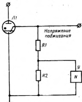
Л1 — испытываемый игнитрон; R1; R2 — резисторы делителя напряжения; У — осциллограф
