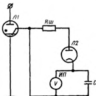
П1 — испытываемый игнитрон; П2 — неонотрон; ИП — вольтметр; С — конденсатор; Rш — резистор
