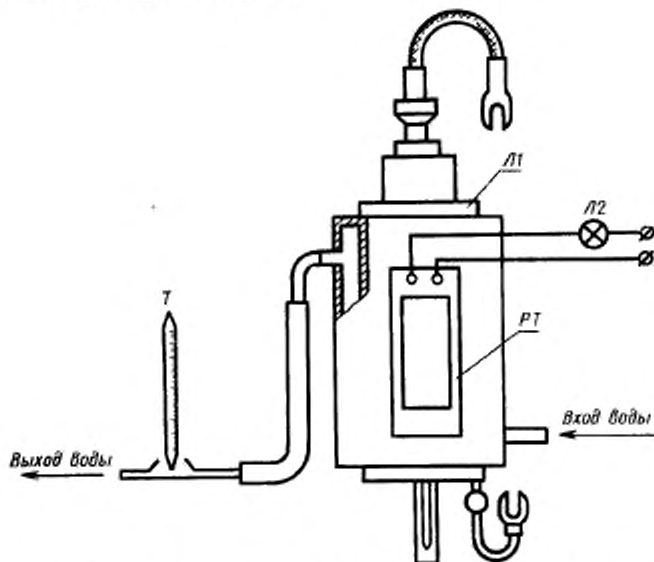
Л1—игнитрон; Л2—сигнальная лампа; РТ—реле тепловой защиты; Т—термометр
