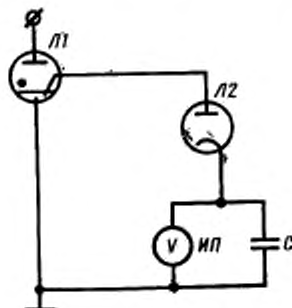
Л1 — испытываемый игнитрон; Л2 — кенотрон; С — конденсатор; ИП — вольтметр
