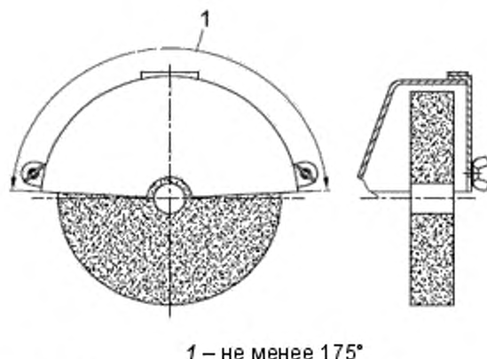
Рисунок D.2 – Защитное ограждение с передним экраном
