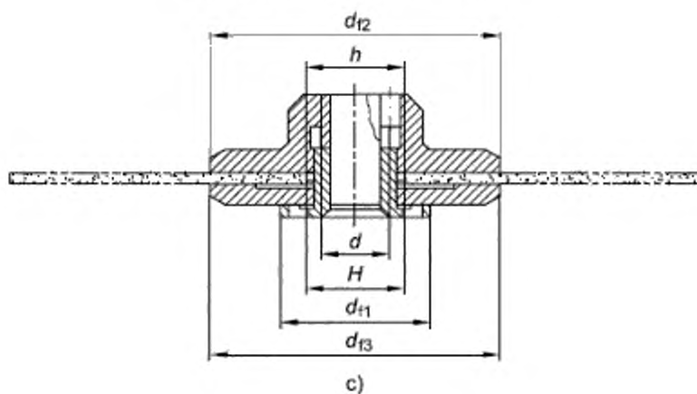
с) Шлифовальный круг типа 41
