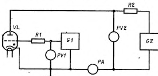
R1, R2 —резисторы; PV1, PV2 —измерители напряжения; PA —измеритель тока; VL —испытываемый тиратрон; G1, G2 —регулируемые источники напряжения
