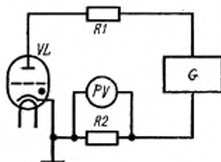
R1 —резистор; R2 —измерительный резистор; PV —измеритель напряжения; VL —испытываемый тиратрон; G —источник напряжения.
