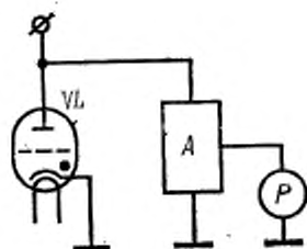
P —осциллограф; VL —испытываемый тиристор; A —делитель напряжения.
