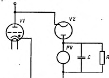
R —резистор; C —конденсатор; PV —измеритель напряжения; V1 —испытываемый тиратрон; V2 —диод
