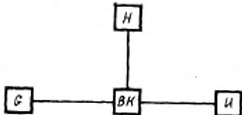
Г—генератор; Н—нагрузка; ВК—выходной контур; И—индикаторное устройство.
