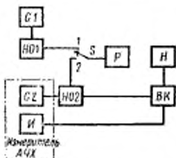
G1 — генератор стандартных сигналов; G2 — генератор качающейся частоты; P — измеритель частоты; S — переключатель; NO1 , NO2 — направленные ответвители; И — индикаторное устройство; BK — выходной контур; Н — нагрузка
