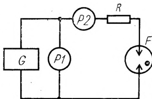
R —защитный резистор; P1 —измеритель напряжения; P2 —измеритель тока; F —испытуемый разрядник; G —источник постоянного напряжения
