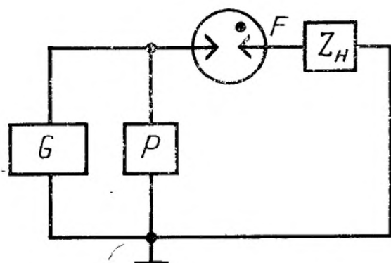
G —источник импульсного напряжения; P —измеритель напряжения; F —испы- тельный разрядник; Z_H —нагрузка или эквивалент нагрузки
