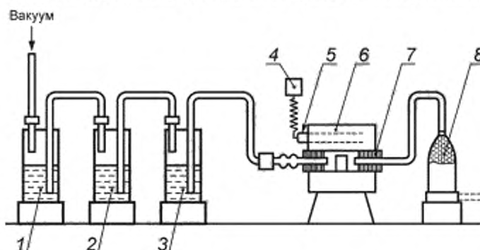
1—3 — склянки Дрекслея поглотительные, 4 — терморегулятор, 5 — термопара; 6 — печь трубчатая электрическая, 7 — лодочки фарфоровые; 8 — склянка Тищенко СРТ
