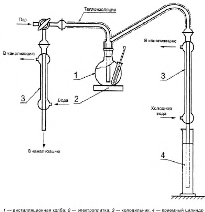
1 — дистилляционная колба; 2 — электроплитка; 3 — холодильник; 4 — приемный цилиндр
